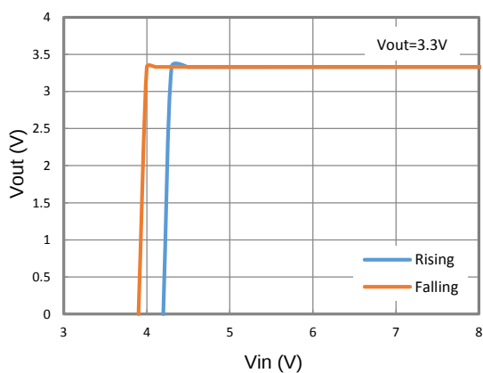
VIN UVLO
