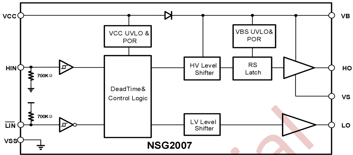
图 10-1 NSG2007 功能框图
