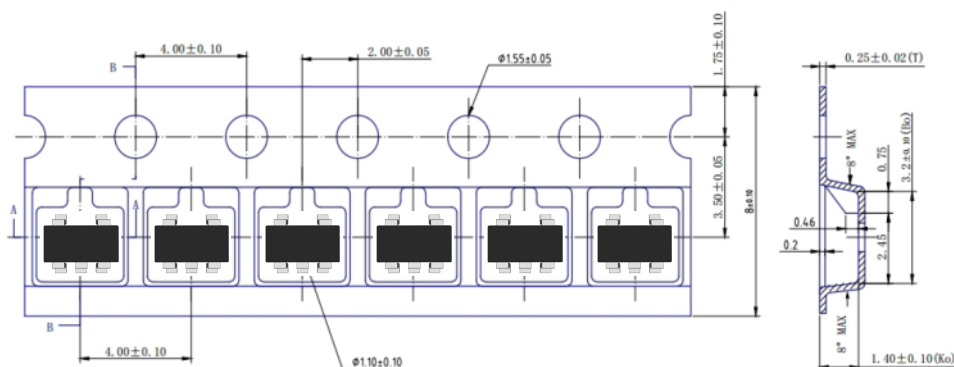
SOT-23-5
