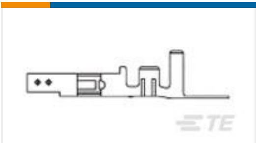
TE Part #794956-4 VAL-U-LOK SKT PHBZ AU 22-18AWG
