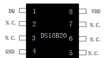
MSOP8
