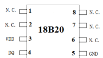
SOP8
