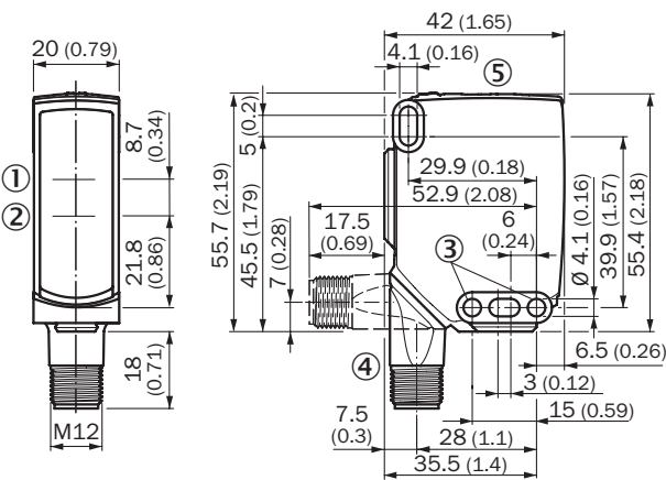
感测器尺寸圖
