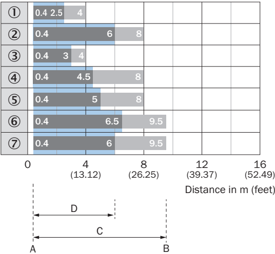
触发感应距离图表
