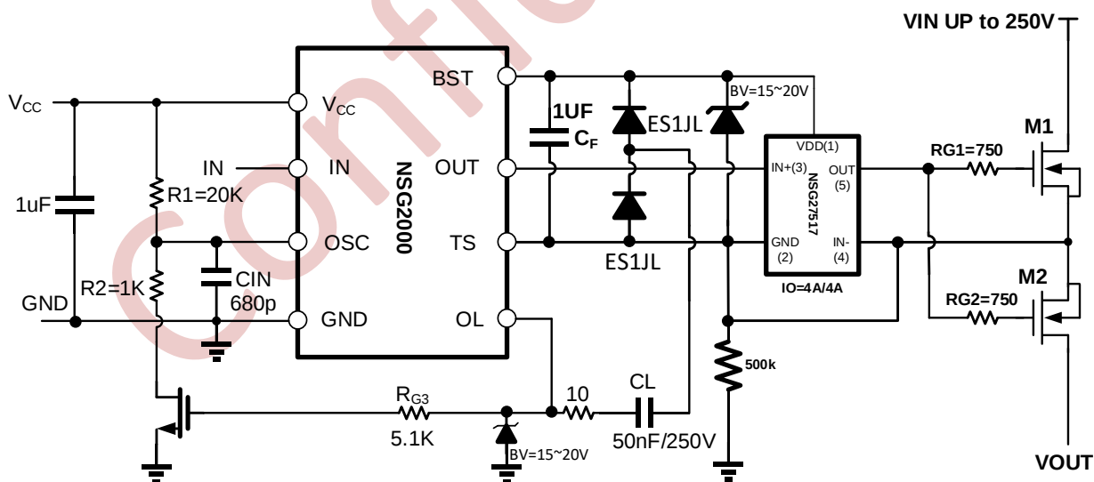
图 10-7 典型应用电路图 6 利用 NSG27517 扩流至 4A/4A 电流能力
