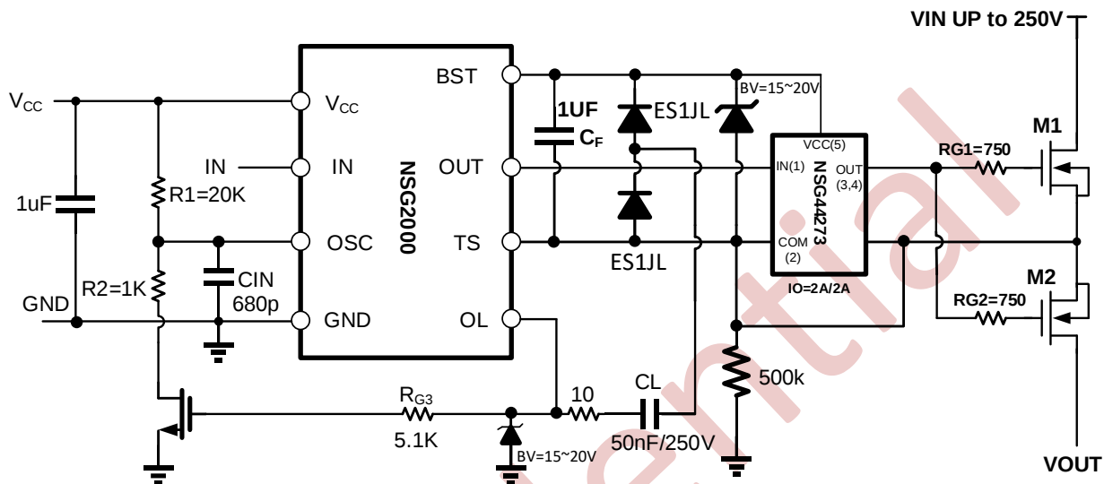
图 10-6 典型应用电路图 5 利用 NSG44273 扩流至 2A/2A 电流能力
