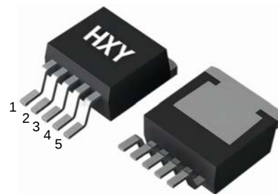
TO-263-5L (TO-263-5)
