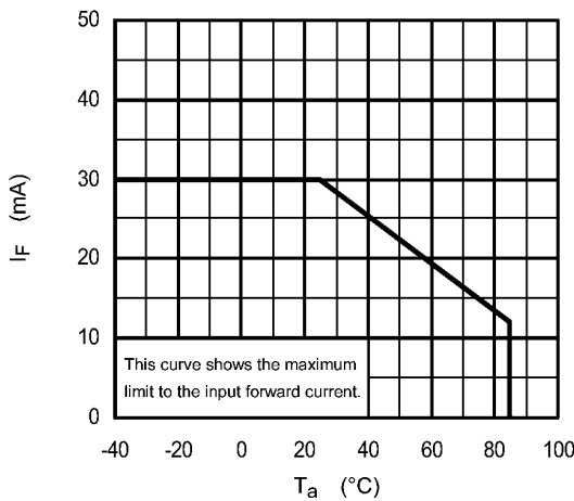
Fig. 13.1.1 I_F - T_a
