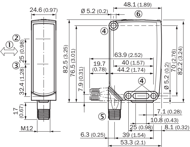
感测器尺寸圖
