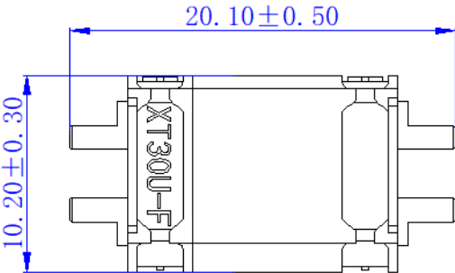
互配尺寸
