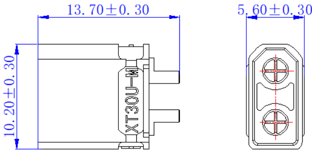
堆叠尺寸
