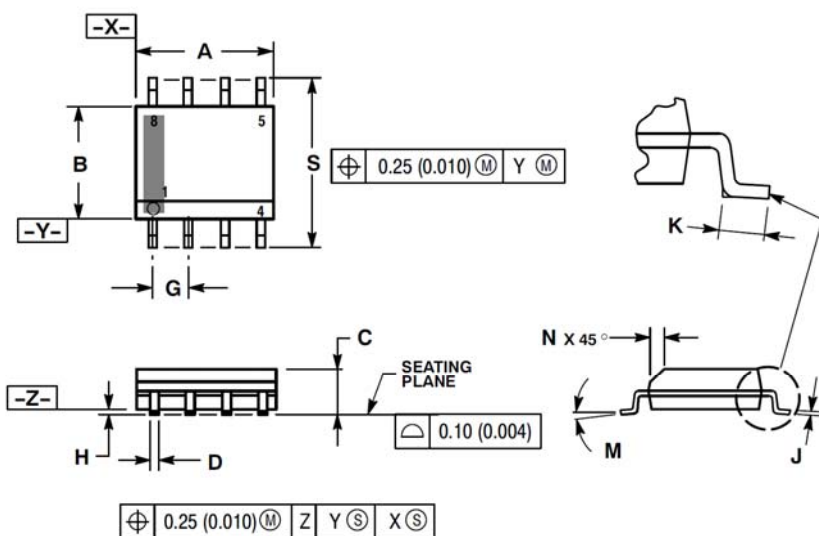
SOP8(SOIC-8)
