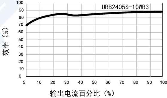
效率 VS 输出负载 (Vin=24V)
