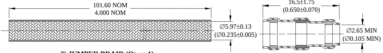
3) SOLDER SLEEVE, Qty.: 2
