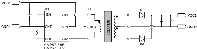
图2. CMP6713RE/CMP6713HV 单路输出
