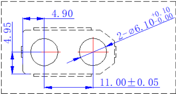
互配尺寸
