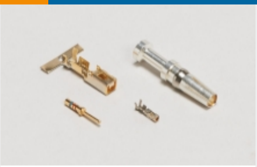
Connector Contacts(64)
