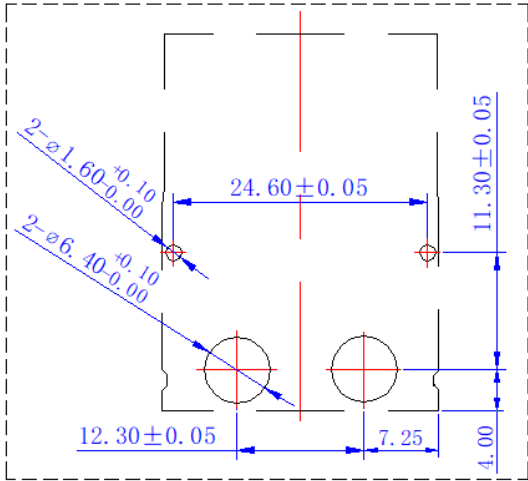
互配尺寸
