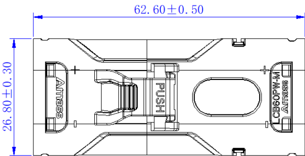
互配尺寸
