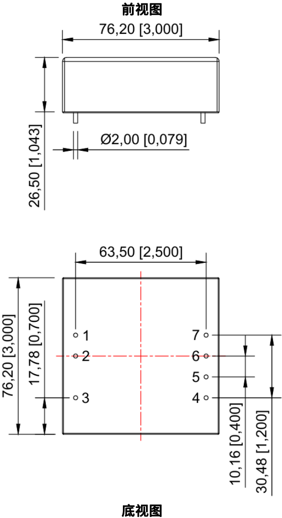
AC220S__DC-80W系列外观尺寸图
