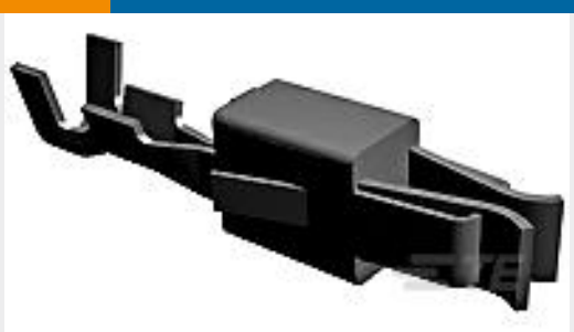
TE Part #927768-9 JPT REC 2.8 Contact SRC Au
