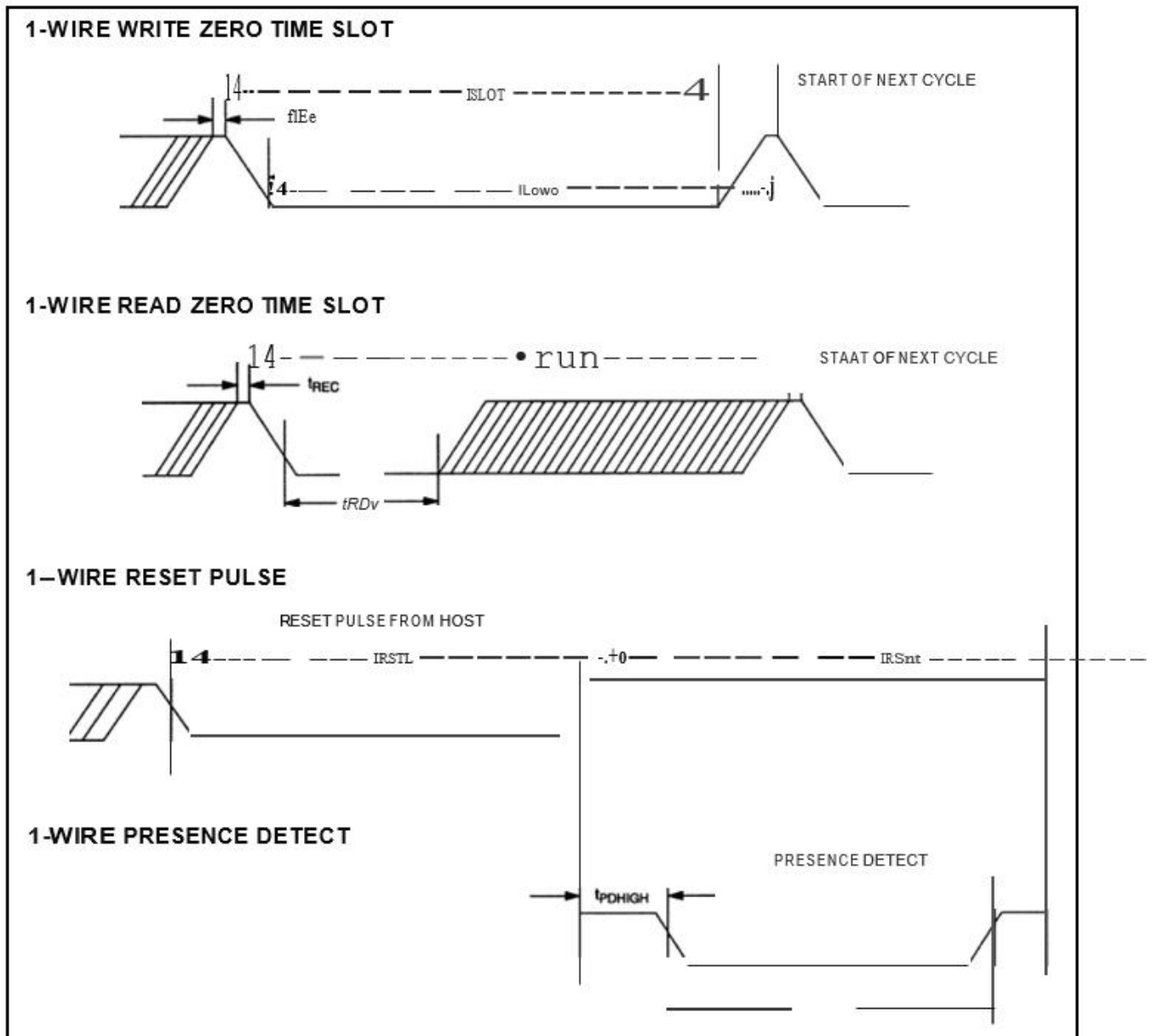
图 18. 时序
