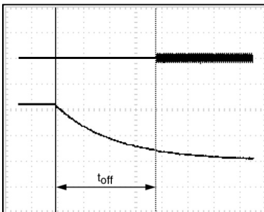
(Abb.6 Detektion Netzausfall T_{\text{off}} )
