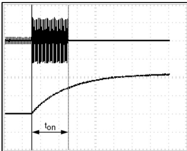
(Abb.5 Begrenzungs-Zeit T_{\text{on}} )
