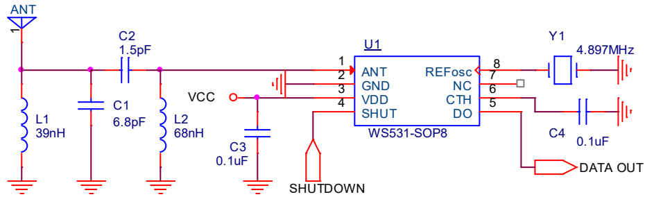
图1 315MHz 3kbps 典型电路
