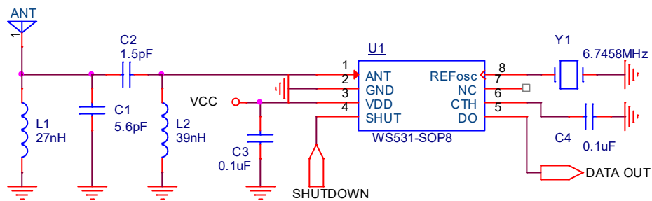
图2 433.92MHz 3kbps 典型电路
