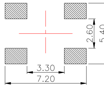
PCB.焊接图
