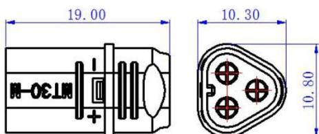
MT30-M
