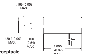
Receptacle
