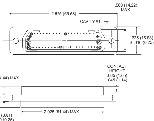
Receptacle
