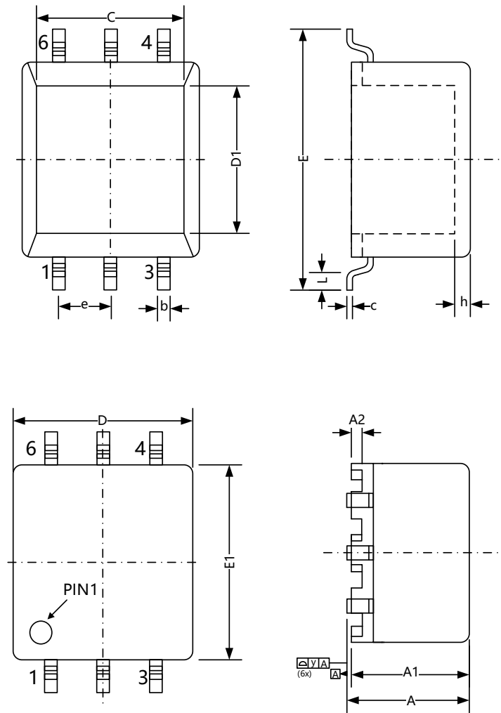
Fig. B.1 SMD-6W 器件外形 (所有尺寸单位为 mm)
