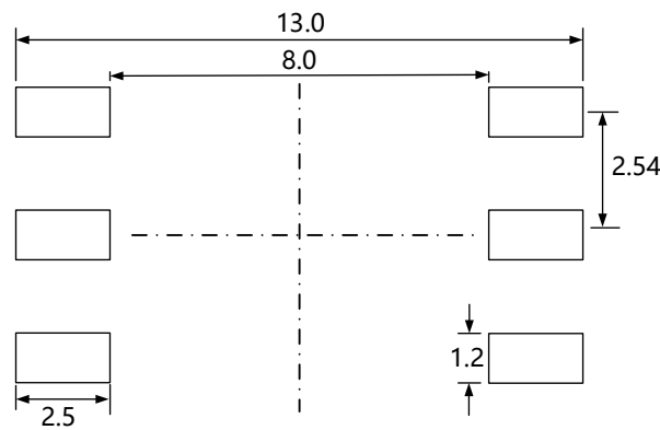
Fig. B.2 SMD-6W 建议焊盘 (所有尺寸单位为 mm)
