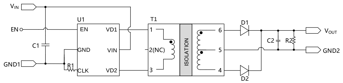
图 9.1 设计原理图
