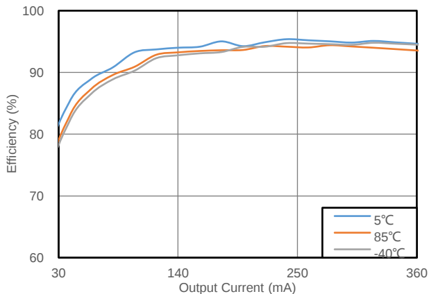
图 8.4 转换效率 vs 输出电流
