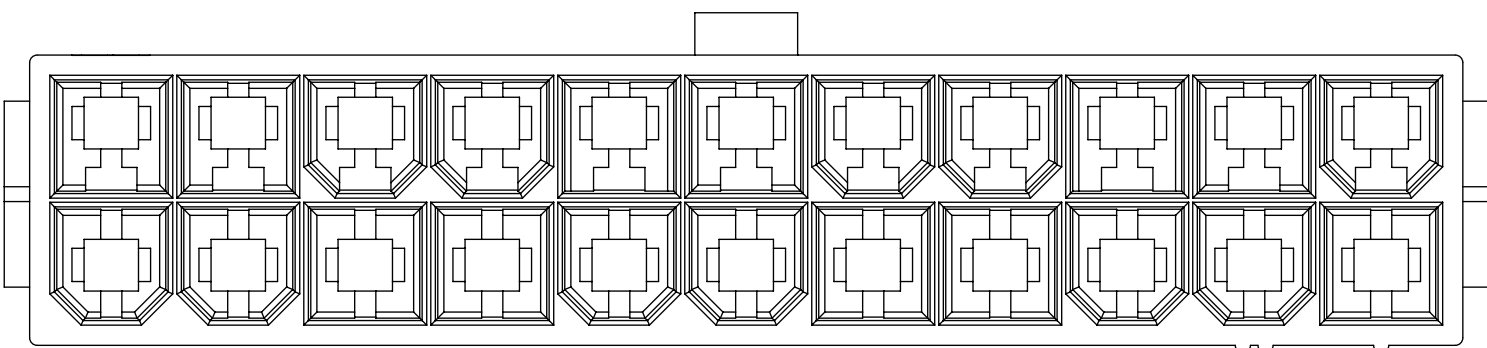
22 CKT
