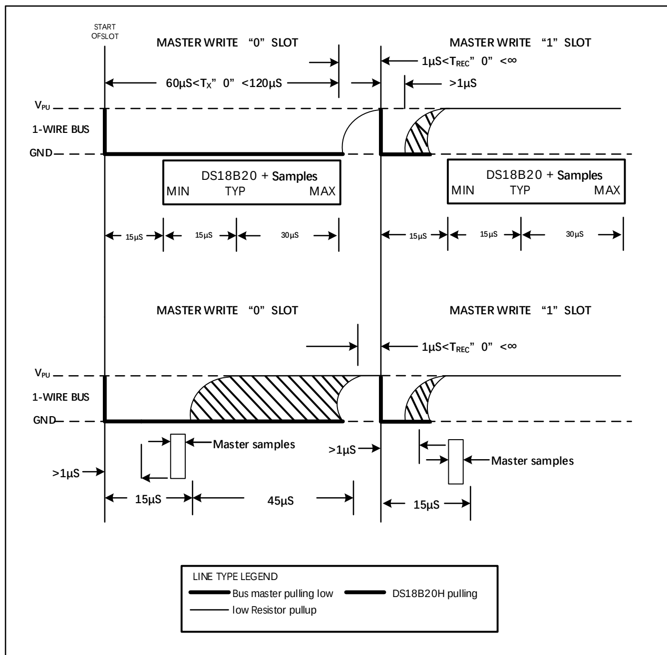
图 14. 读/写时序图
