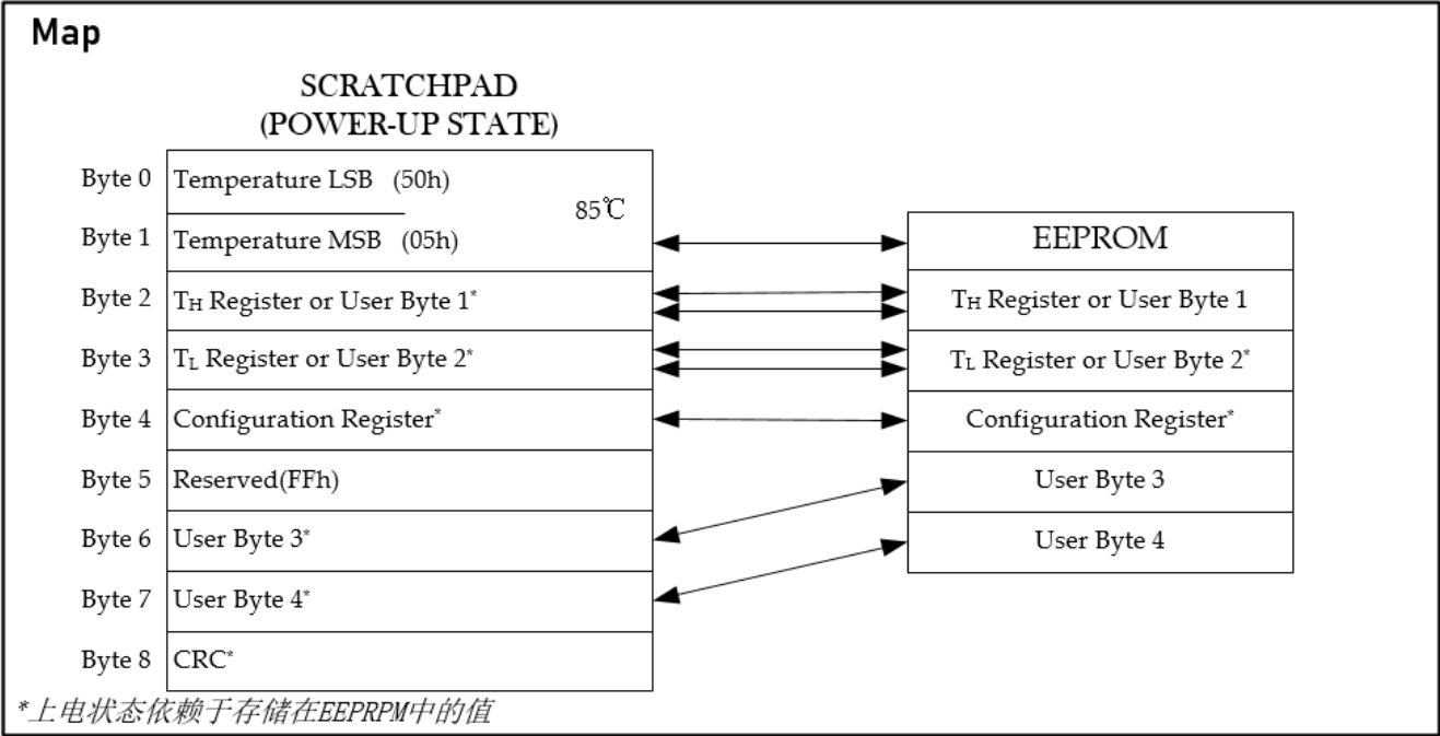
图 7.DS18B20+ 存储器图
