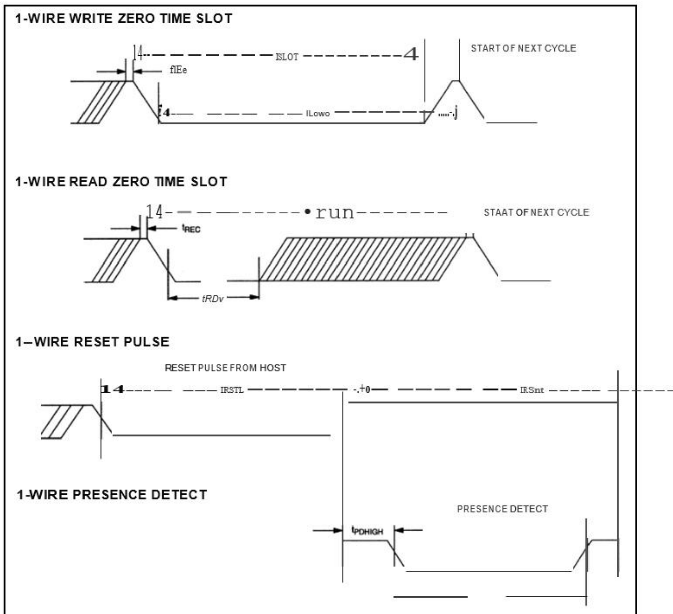
图 18. 时序
