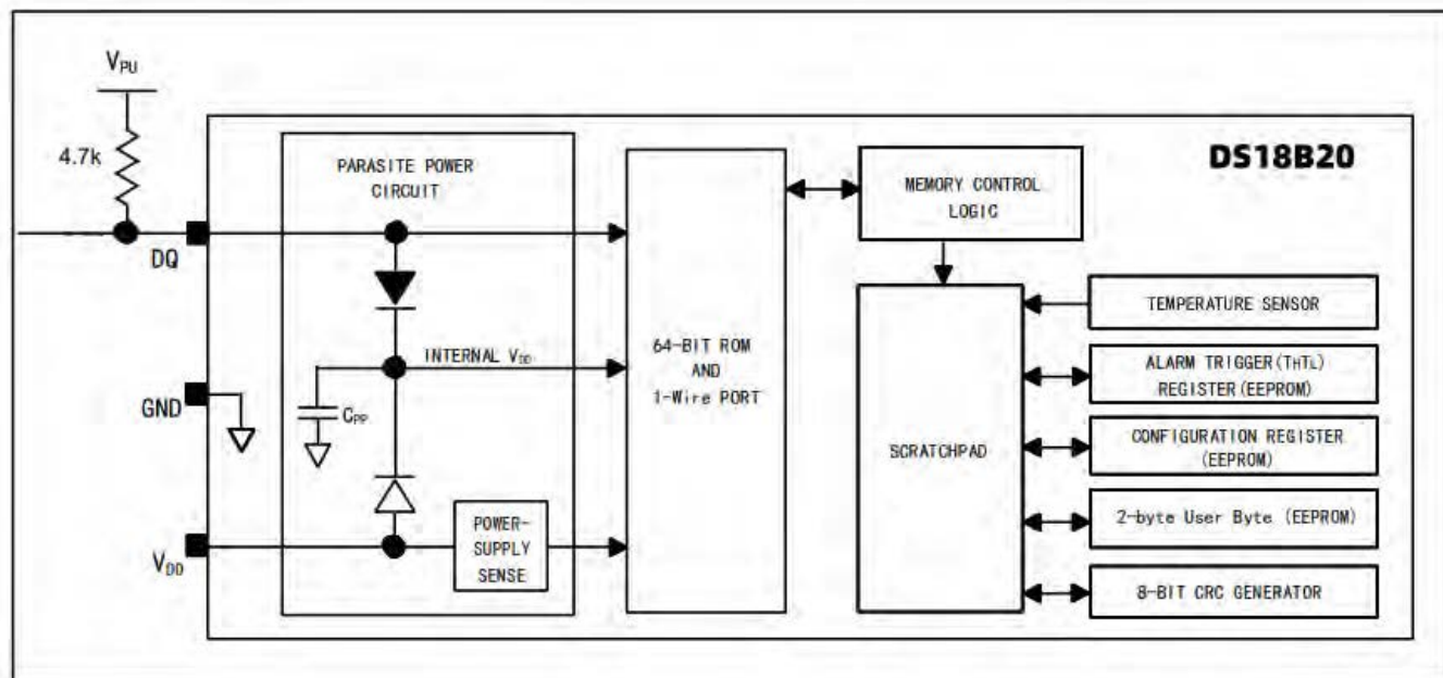
图 1.DS18B20+ 结构框图
