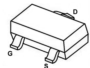
SOT-23-3L
