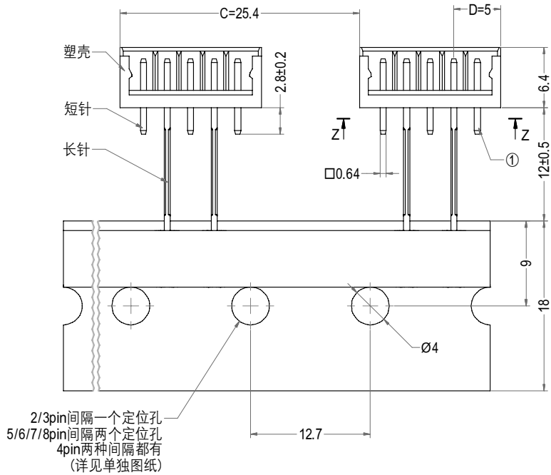
EHB-5AC(2.4长针)编带装
