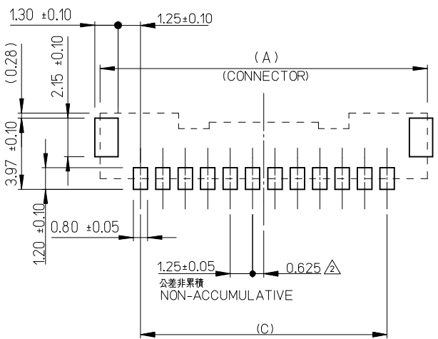
推奨基板レイアウト RECCOMENDED PCB PATTERN LAYOUT
