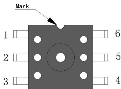
图 1. 引脚定义示意图
