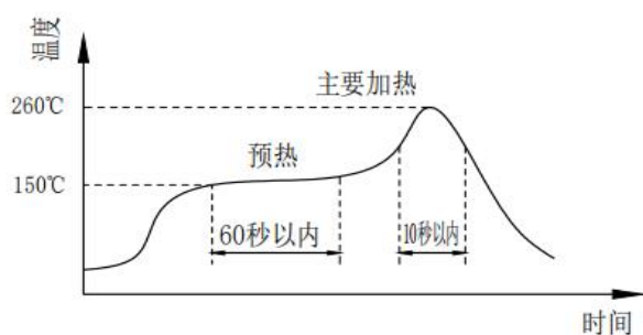
图 13.回流焊接
