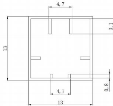
图 7.料管截面示意图
