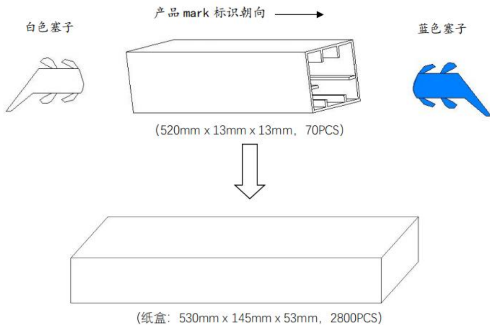
图 15.料管图纸
