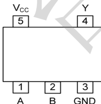
SOT353
