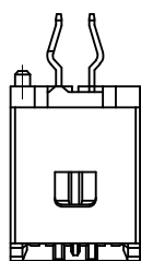
2~3 極形状 ( ロック面及び反ロック面 ) FIGURE OF 2-3 CIRCUIT (LOOK SIDE AND UN-LOCK SIDE)
