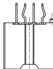
4~5 極形状 ( ロック面及び反ロック面 ) FIGURE OF 4-5 CIRCUIT (LOOK SIDE AND UN-LOCK SIDE)
