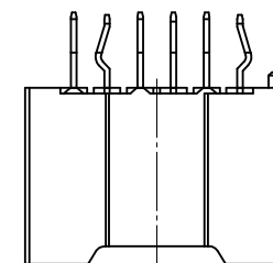
6~7 極形状 ( ロック面及び反ロック面 ) FIGURE OF 6-7 CIRCUIT (LOOK SIDE AND UN-LOCK SIDE)
