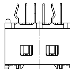
6~7 極形状 ( ロック面及び反ロック面 ) FIGURE OF 6-7 CIRCUIT (LOOK SIDE AND UN-LOCK SIDE)
