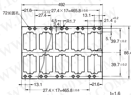
PYP-36
