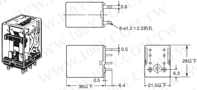
MY2J
