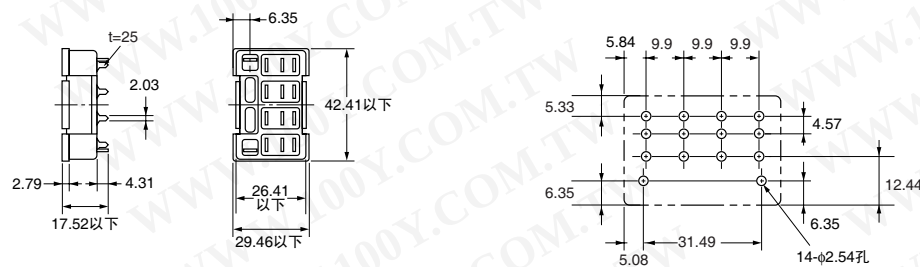
端子排列与类 型PT14相同
