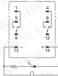
MY2J-CR
