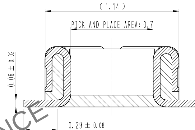
A-A (50:1)
