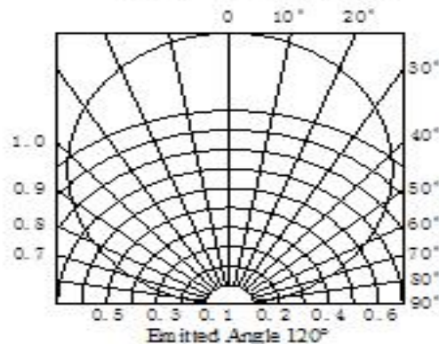
成品发光角度
