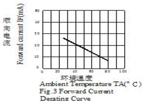
电流与环境温度关系
