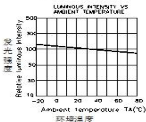
环境亮度 发光强度与环境温度关系
