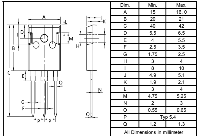
T0-247
