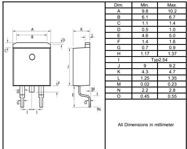
T0-263C
