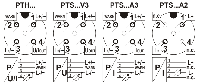
Abb. 3. A-codierter M12-Stecker
