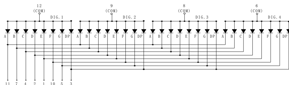
KW4-311CGA
