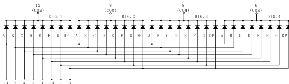
KW4-311CGA
