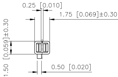
SEC:D-D
