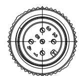
Conn.1
