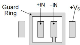
Figure4. Useaguardringaroundsensitvepins
