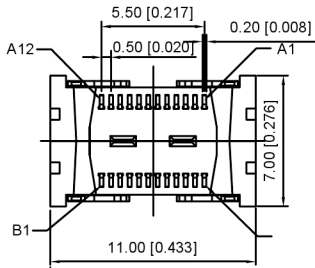
(COVER 尺寸)
