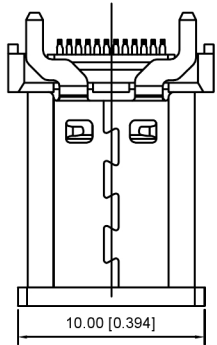
(COVER 尺寸)
