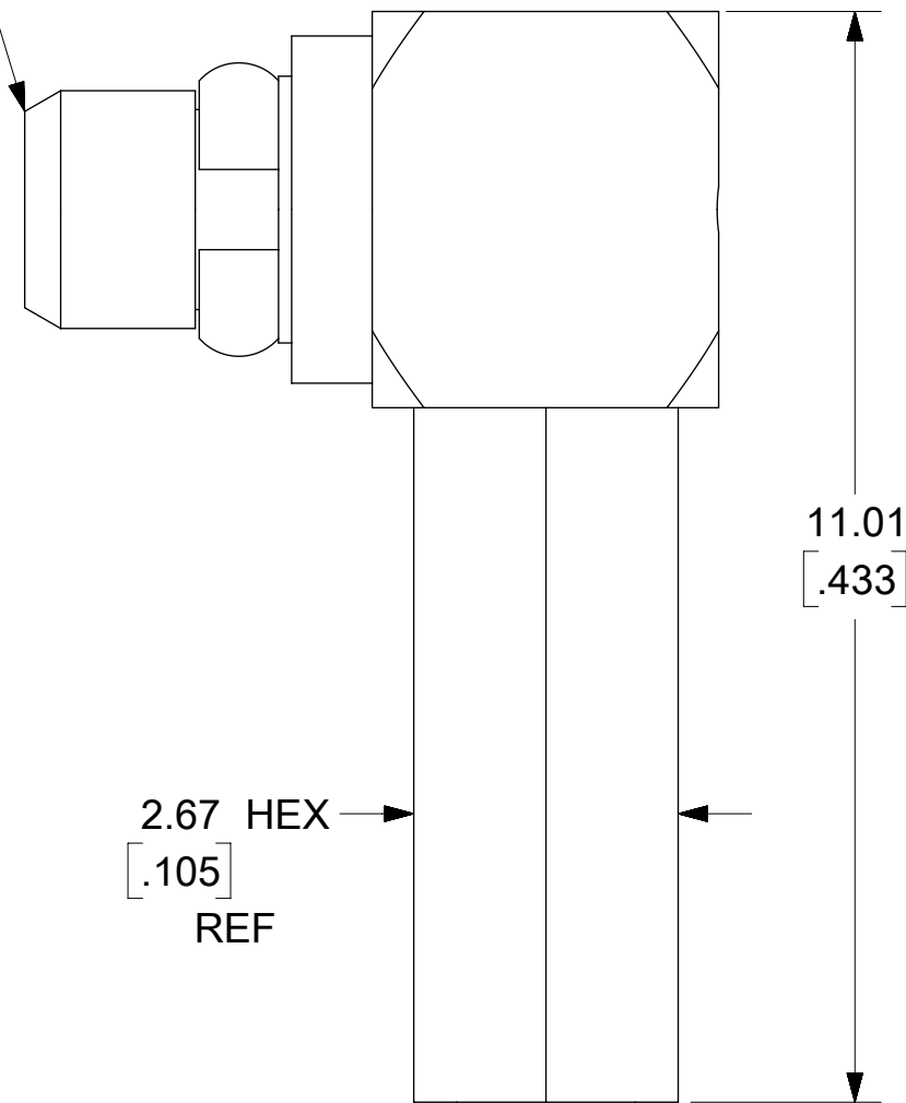
RG178 CABLE
