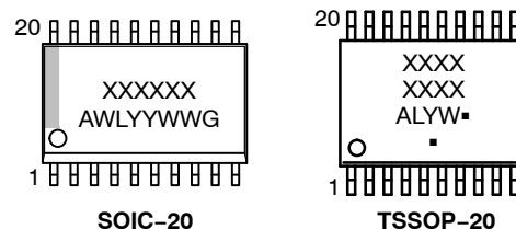
SOIC-20
