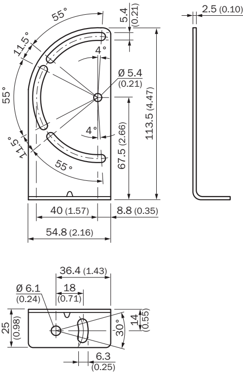
尺寸图 (尺寸单位: mm)
