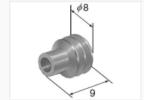
4.8mm 7165-0131
