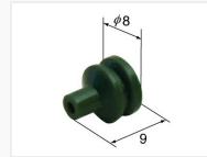
4.8mm 7165-0147
