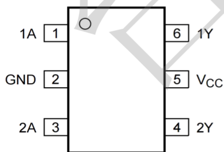
SOT363
